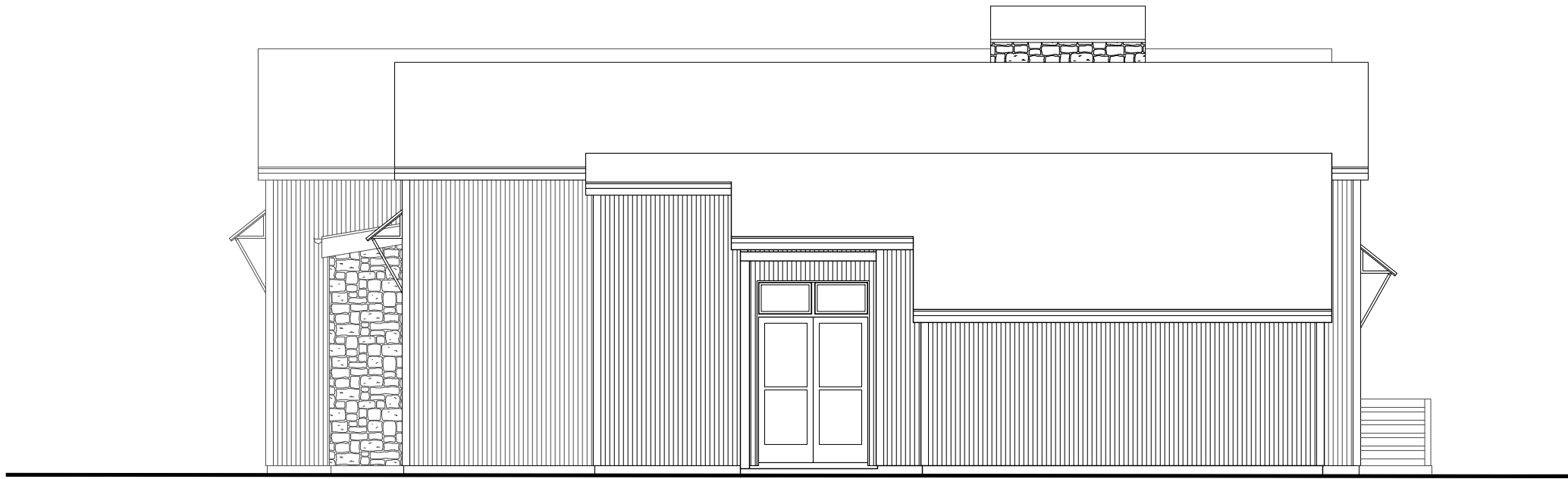
Right Elevation
